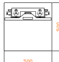
ベース部
