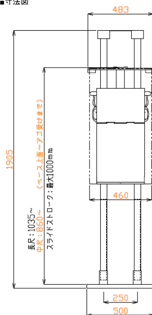
■寸法図
