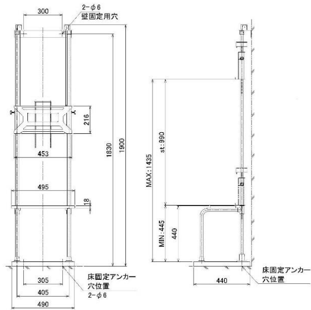
外形寸法図
